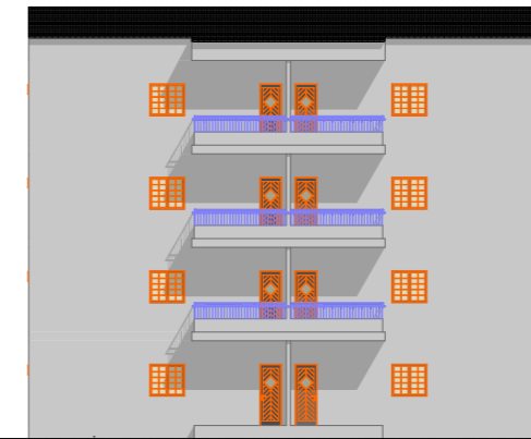
FACADE LATERALE DROITE
