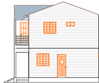
PLAN DE FACADE LATERALE DROITE
